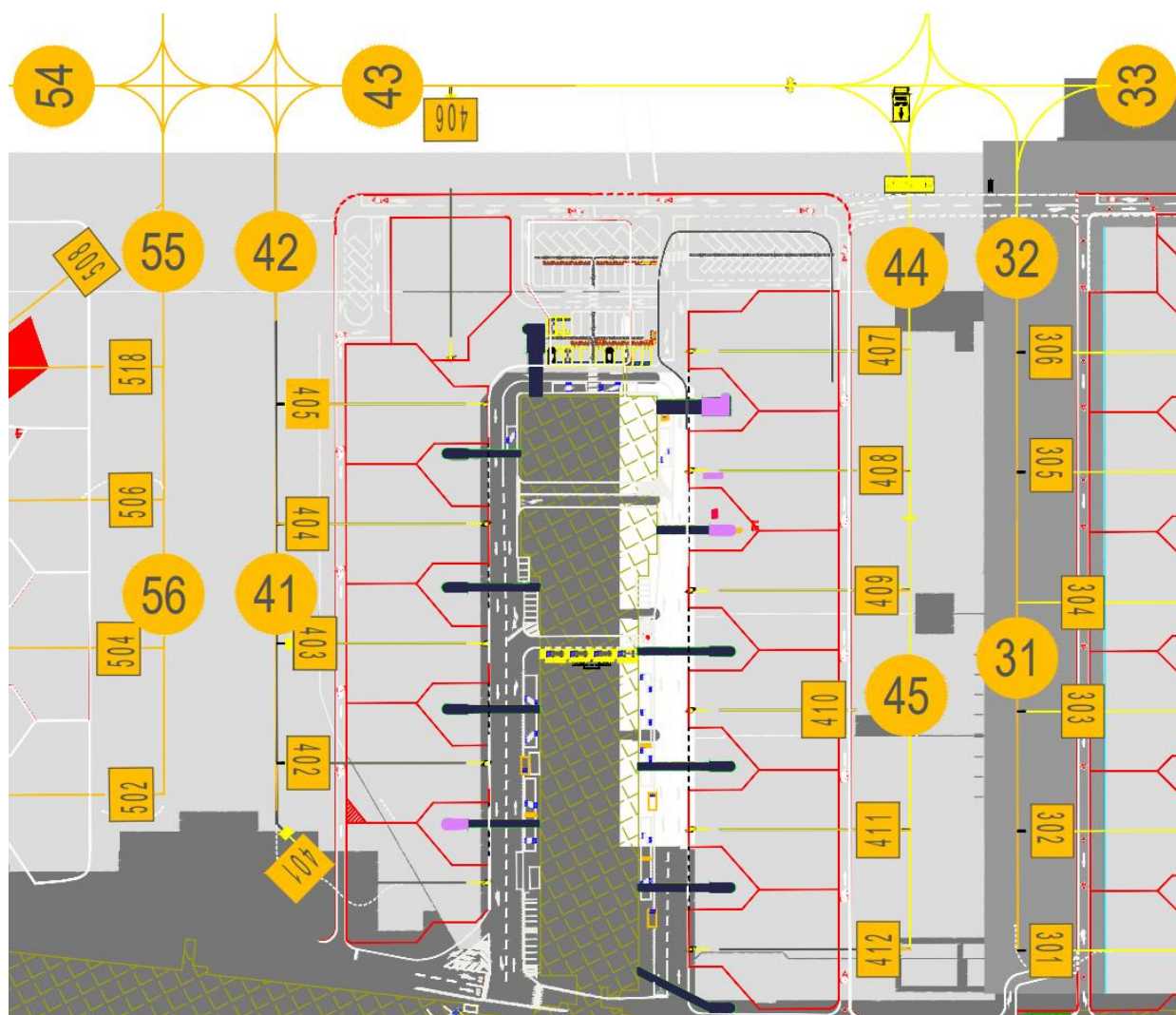
Figura 17. Pista 25 – Partenze piazzali 400
