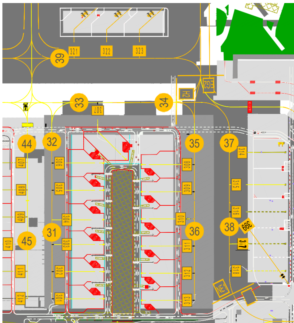
Figura 16. Pista 25 - Partenze piazzali 300
