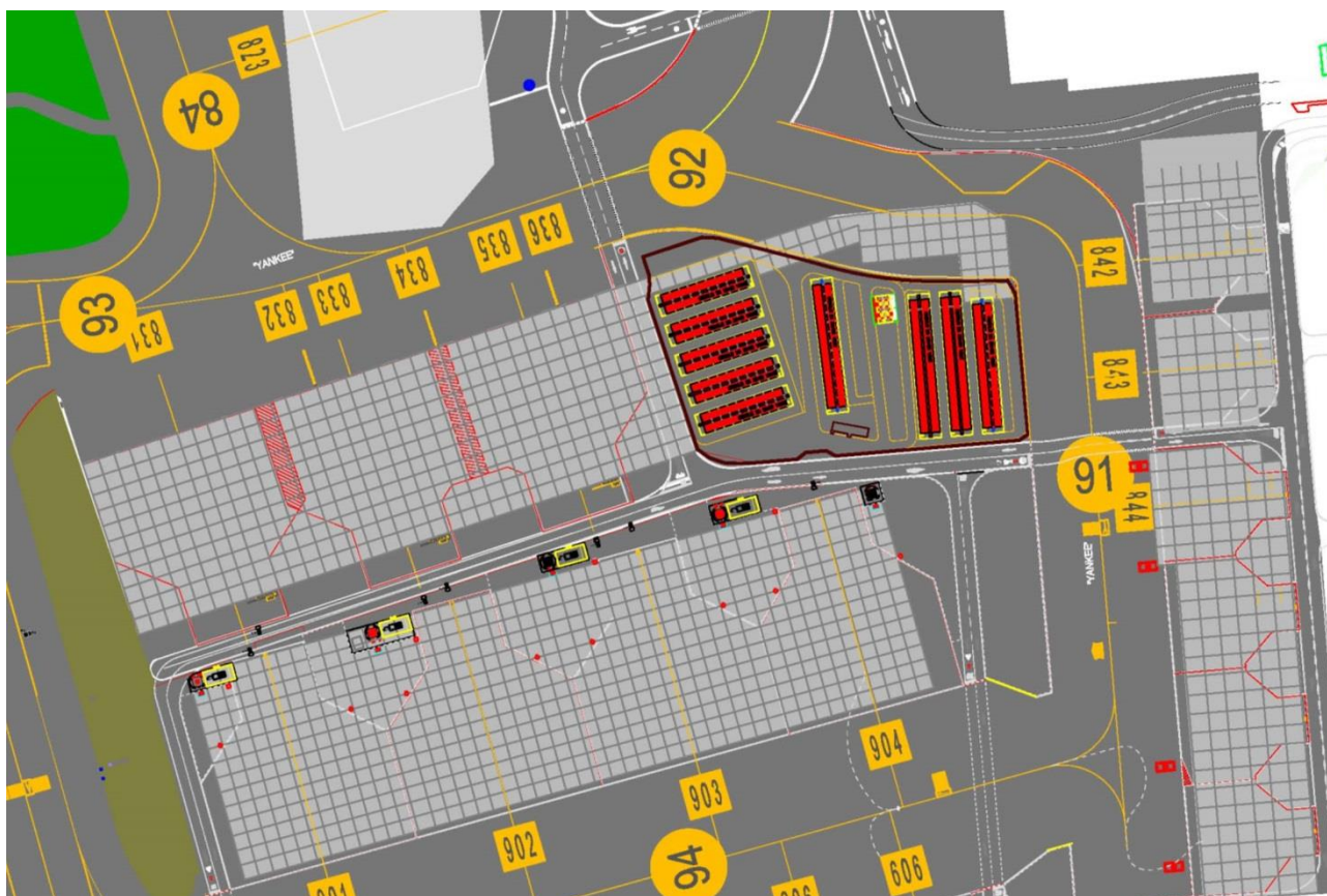
Figura 12. Pista 16L/34R- Arrivi piazzali 800 (da 831 a 845)
