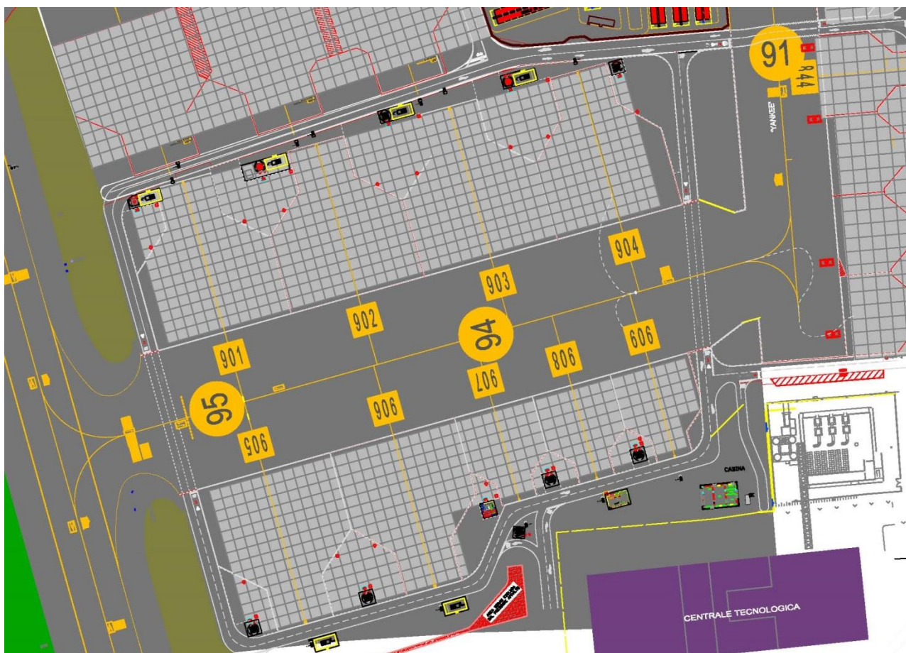
Figura 13. Pista 16L/34R - Arrivi piazzali 900
