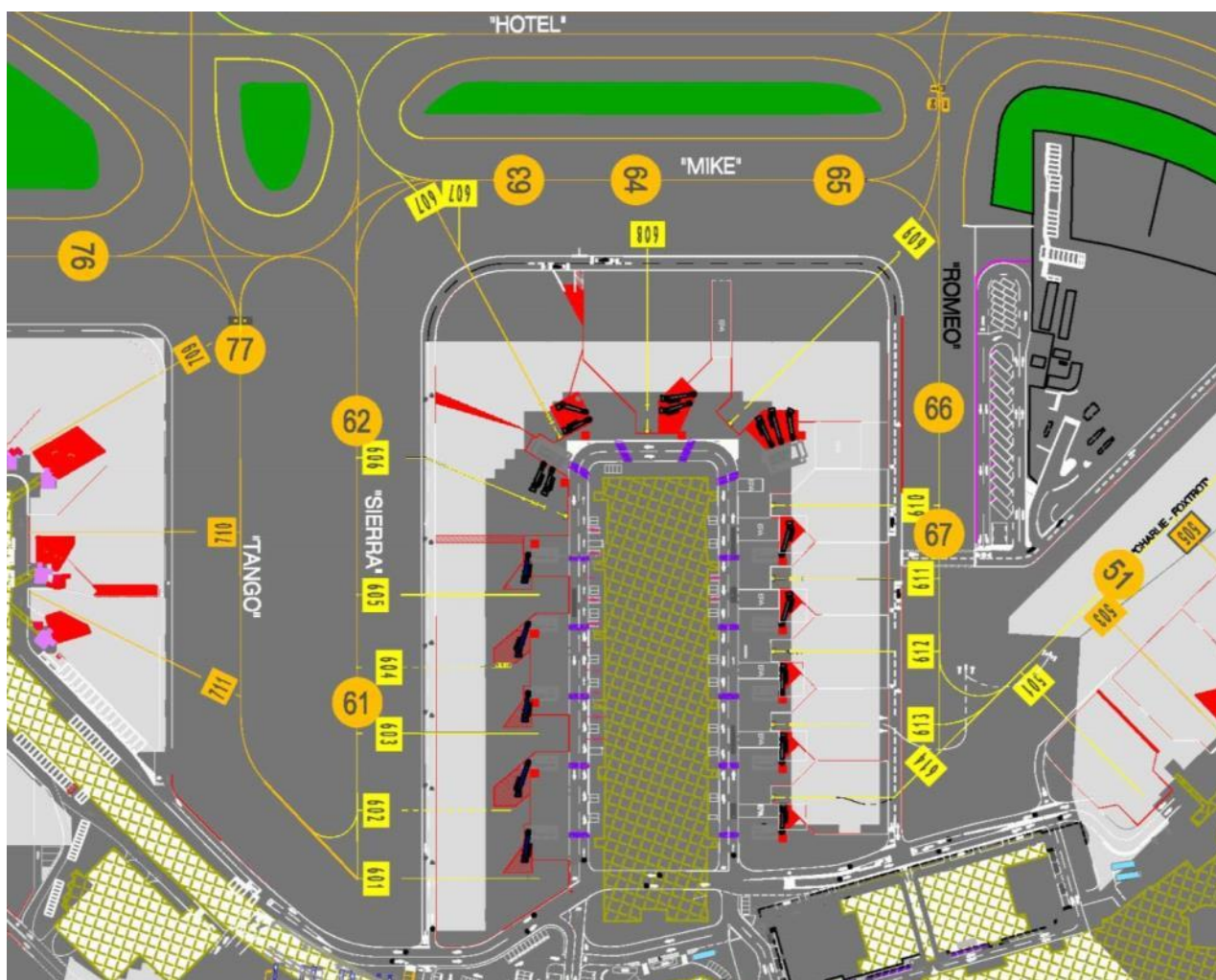
Figura 9. Pista 16L/34R - Arrivi piazzali serie 600
