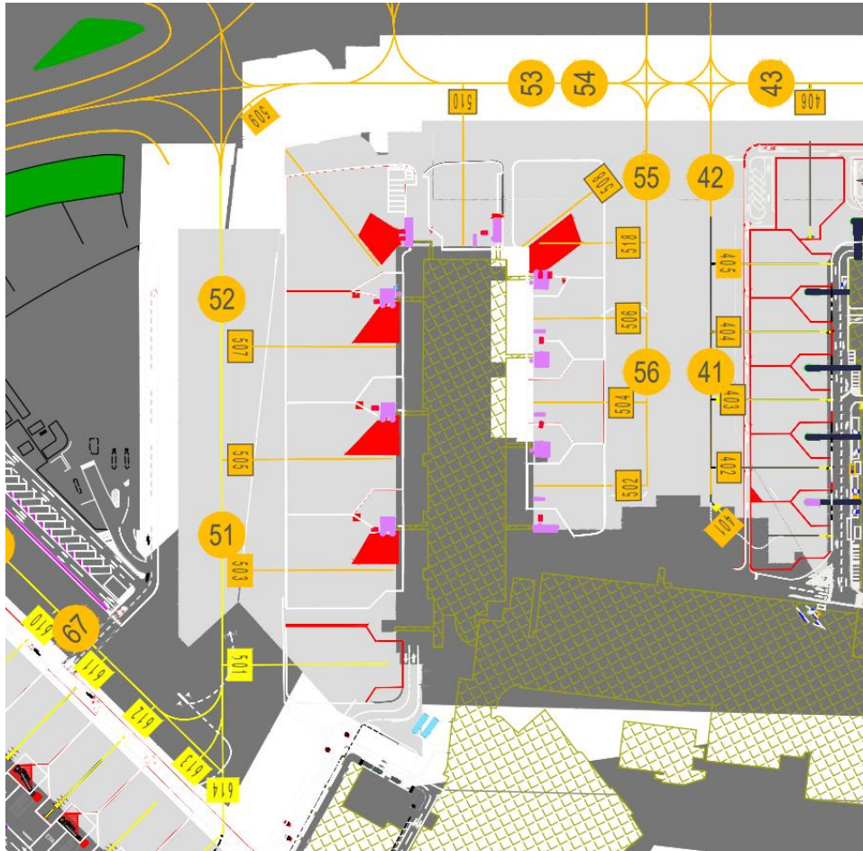
Figura 8. Pista 16L/34R- Arrivi piazzali serie 500
