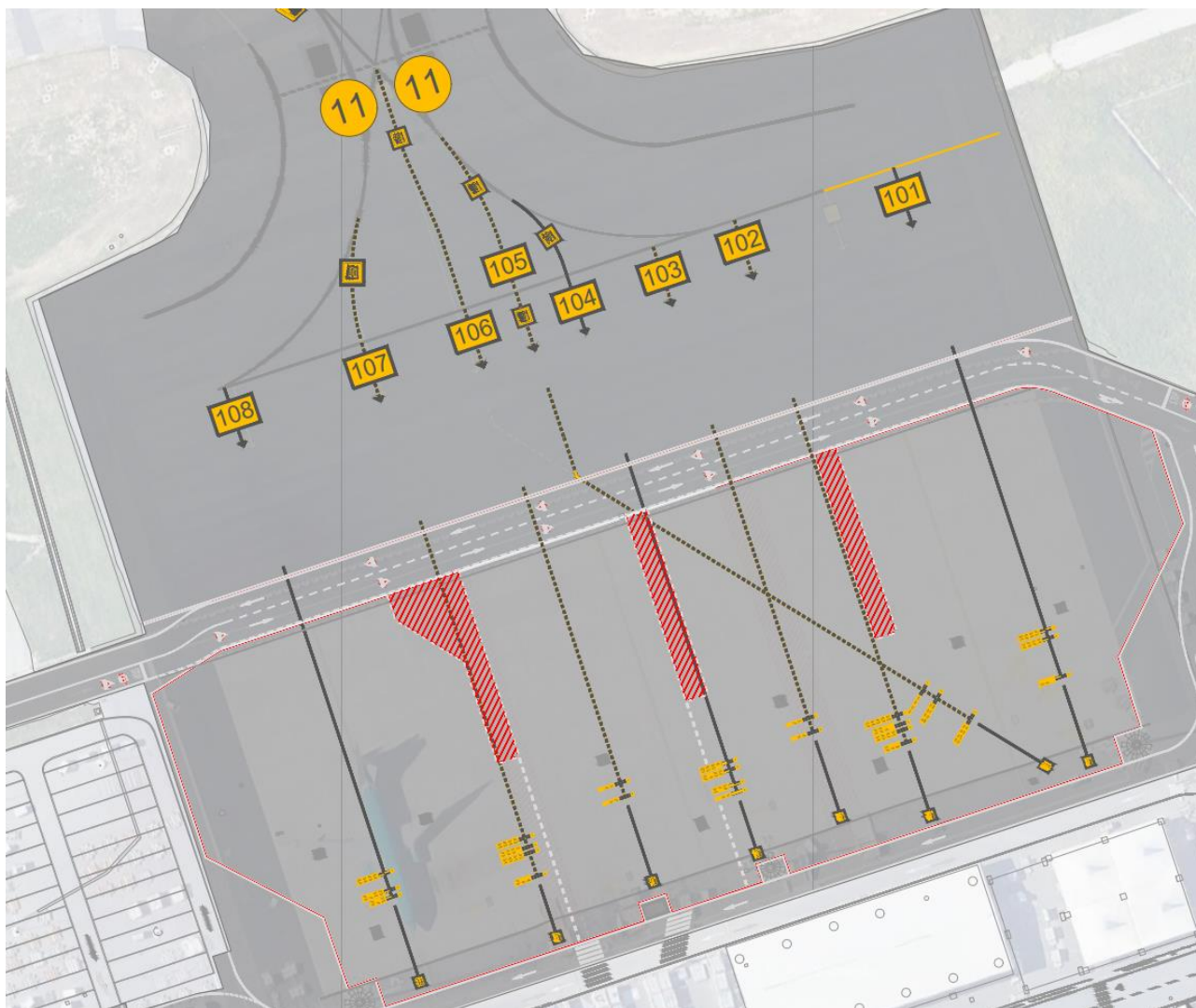
Figura 4. Pista 16L/34R - Arrivi piazzali serie 100
