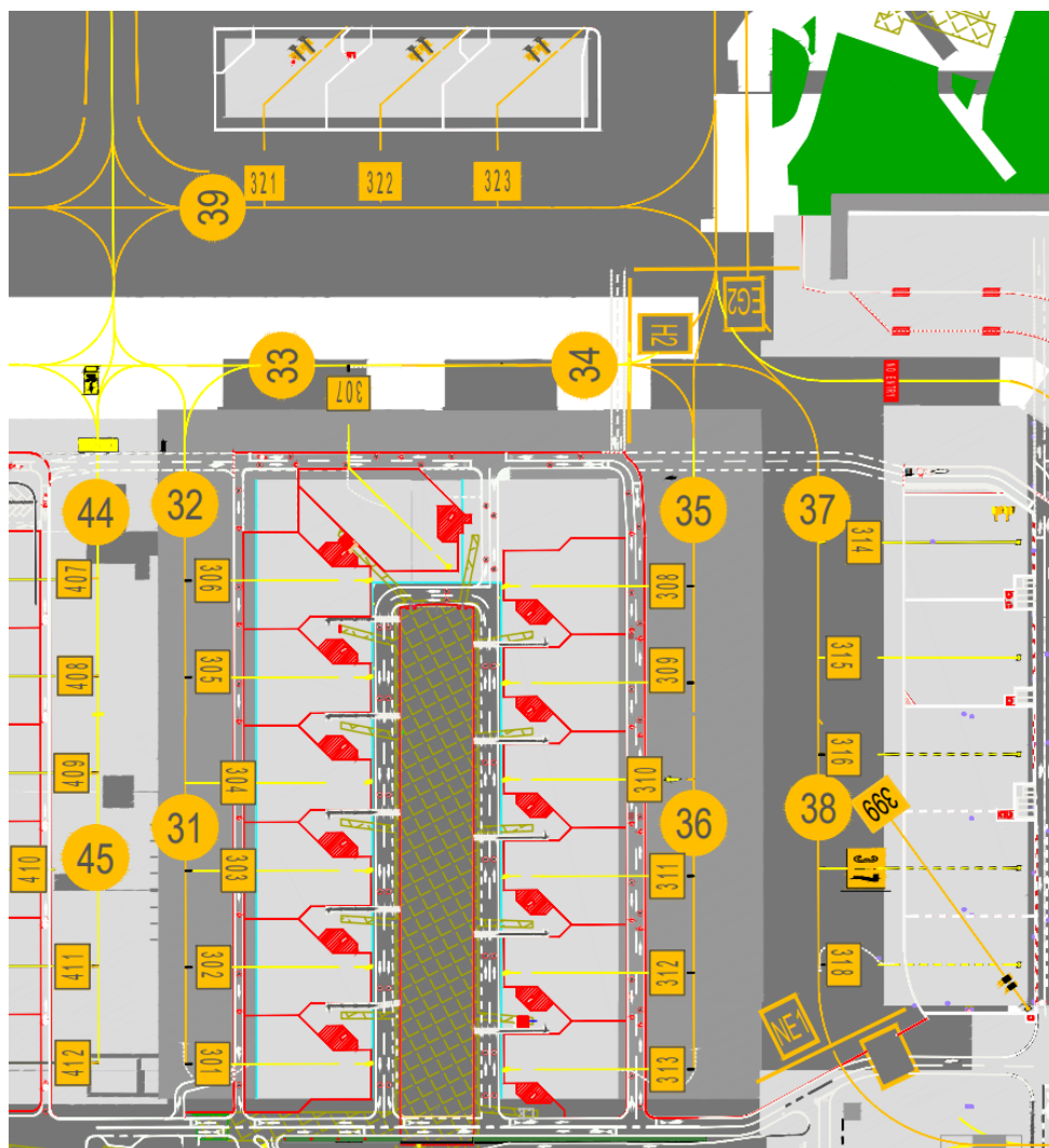
Figura 6 Pista 16L/34R - Arrivi piazzali serie 300
