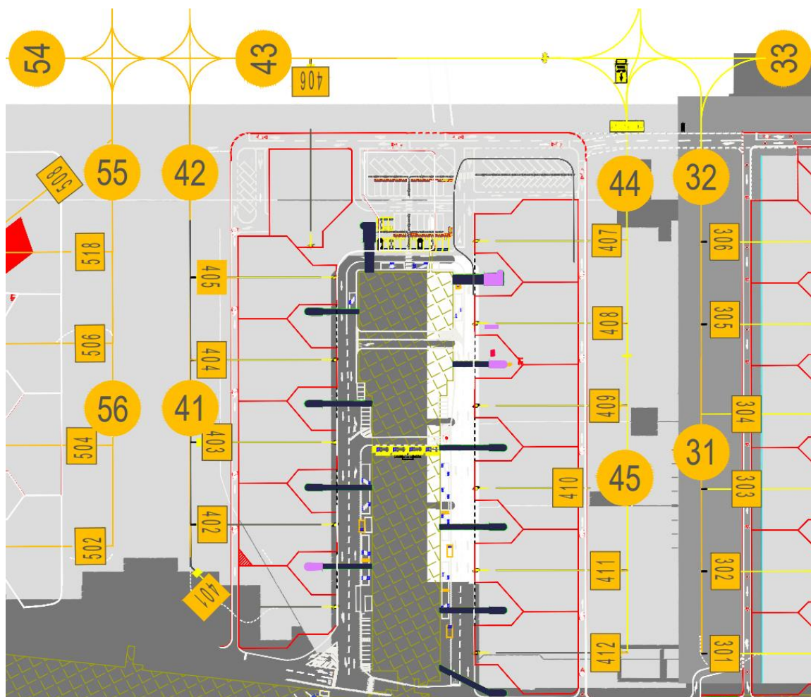
Figura 7. Pista 16L/34R - Arrivi piazzali 400
