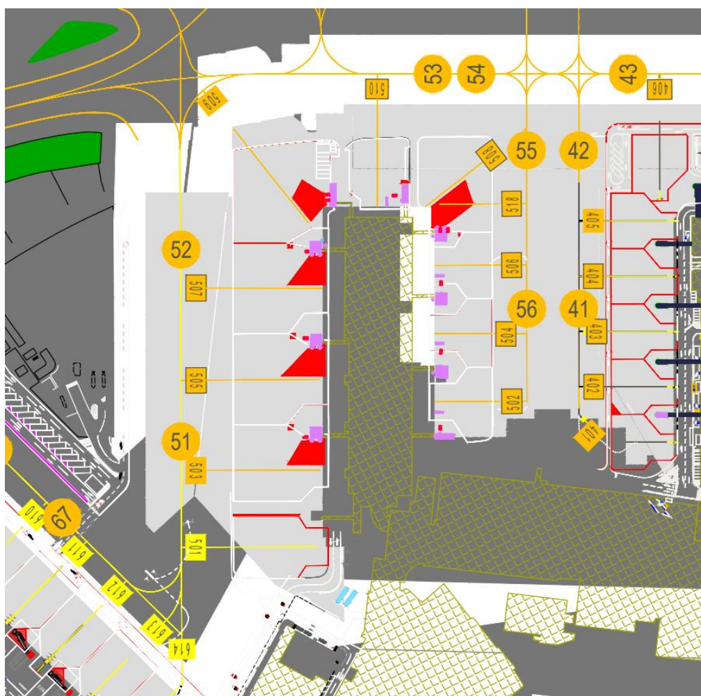
Figura 18. Pista 25 - Partenze piazzali 500
