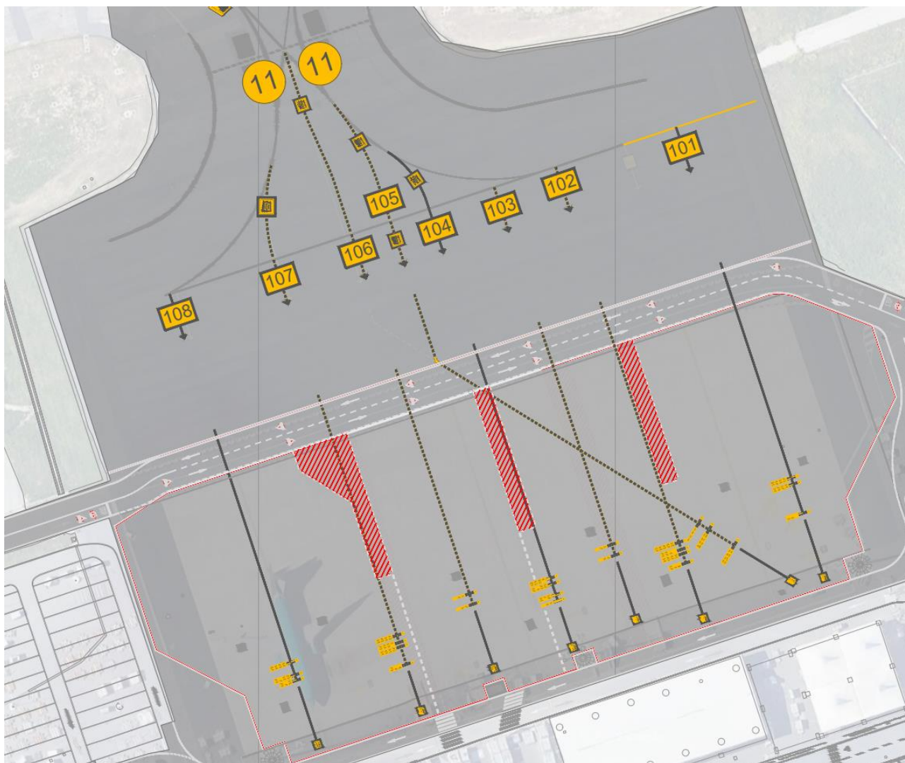
Figura 14. Partenze pista 25 piazzali serie 100
